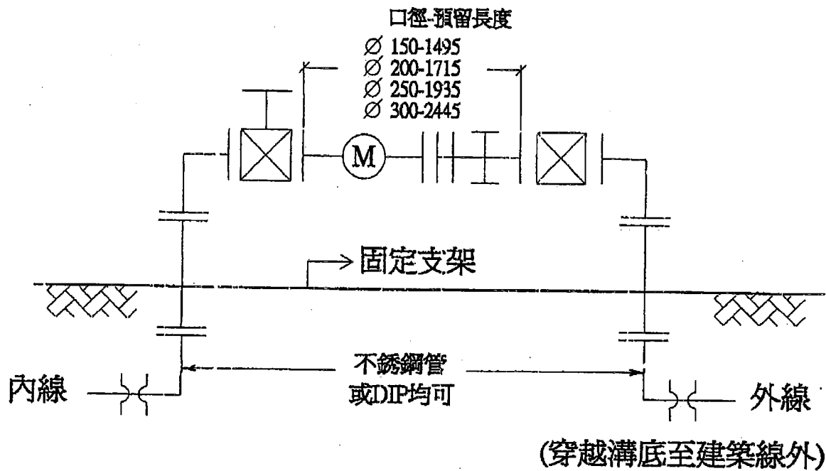
φ 150m/m(含)以上水量計地上式水表組按裝組合參考尺寸示意圖
