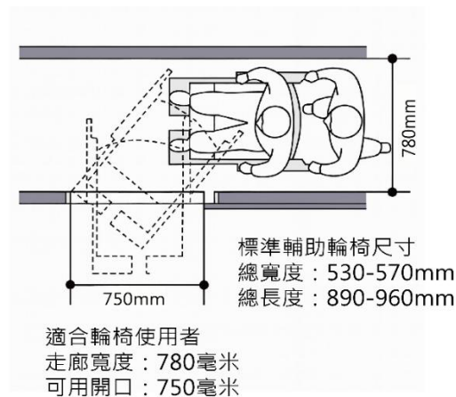
圖 3-9 配件開口的有效尺寸
