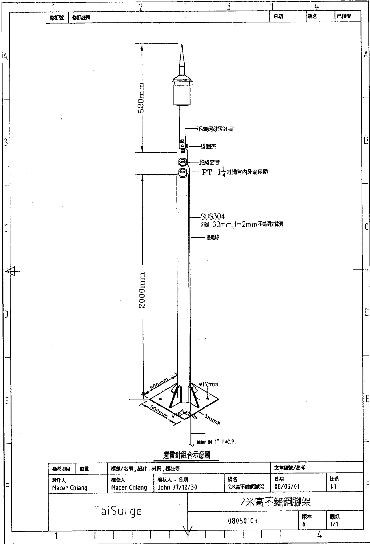
避雷針安裝示意工程圖 2
