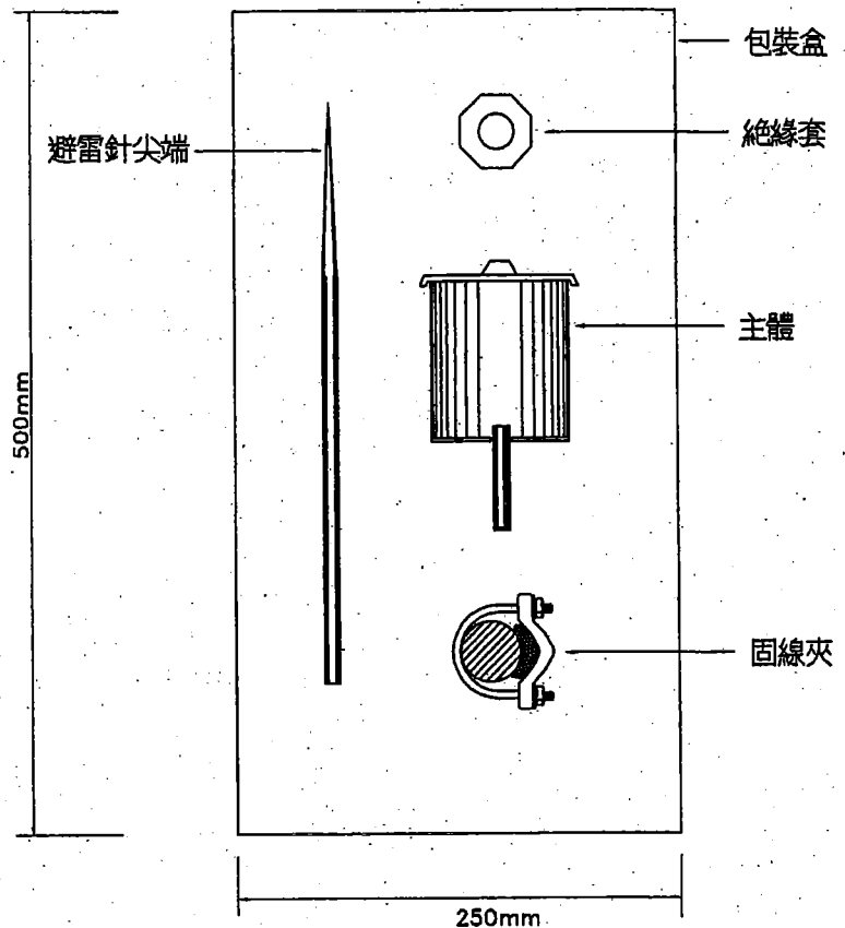
裝箱圖
