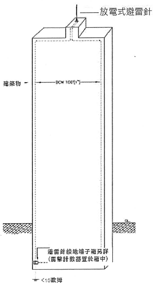
放電式避雷針裝置配線圖
