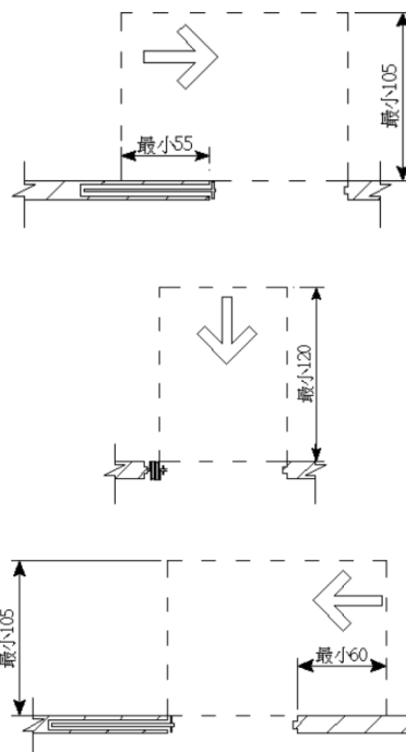
圖 205.2.4.1 推拉門操作空間
