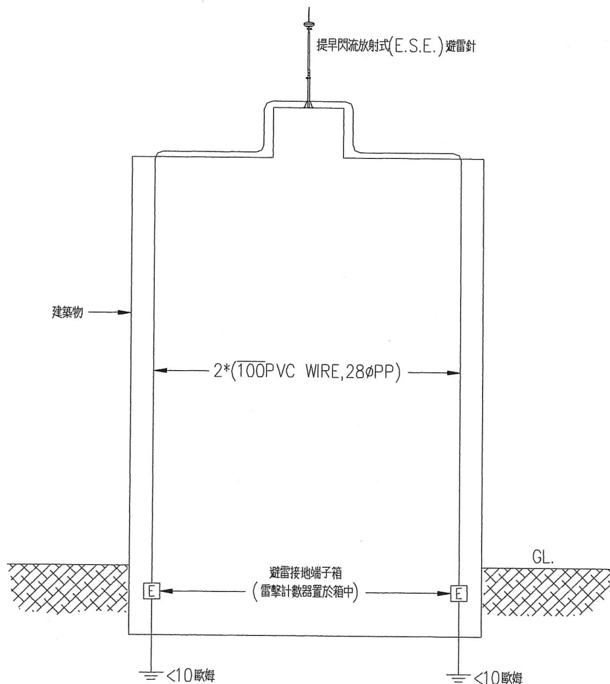
放電式避雷針裝置架構圖（一）
